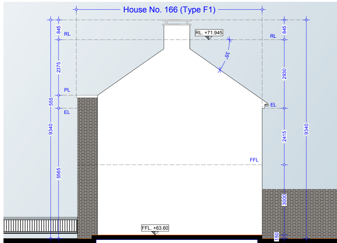
Side Elevation 02 - House Type F1
