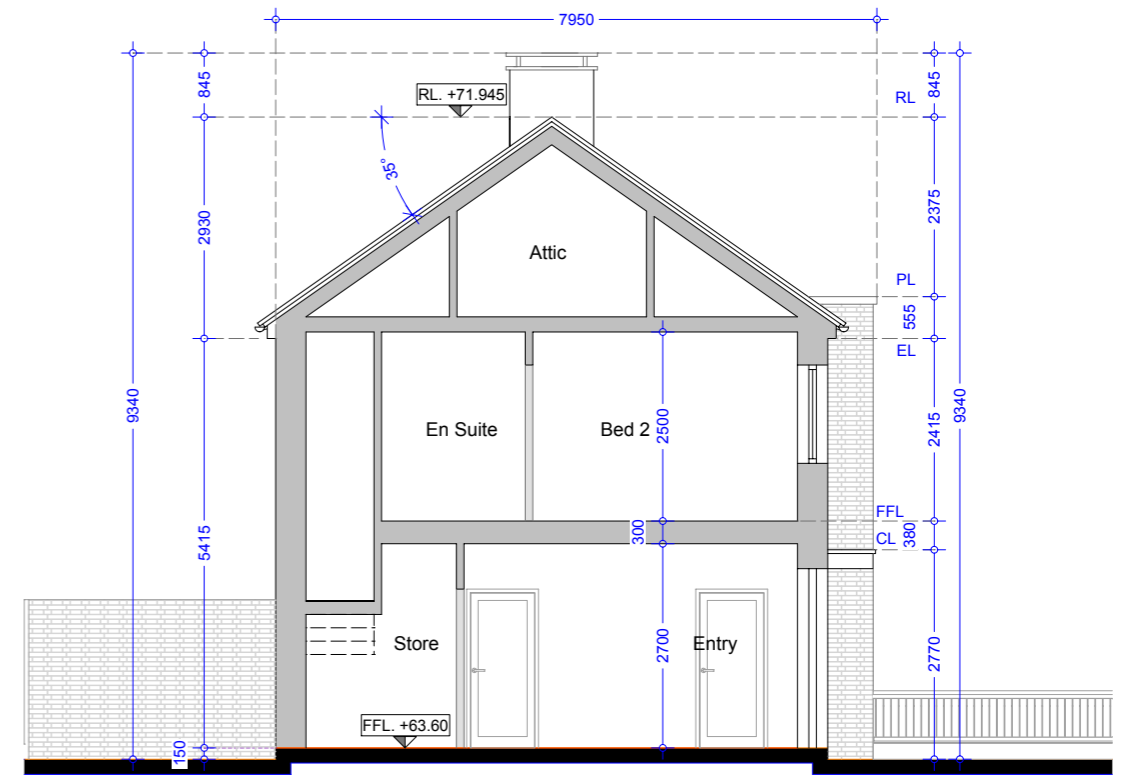
Section AA - House No. 166 - Type F1
