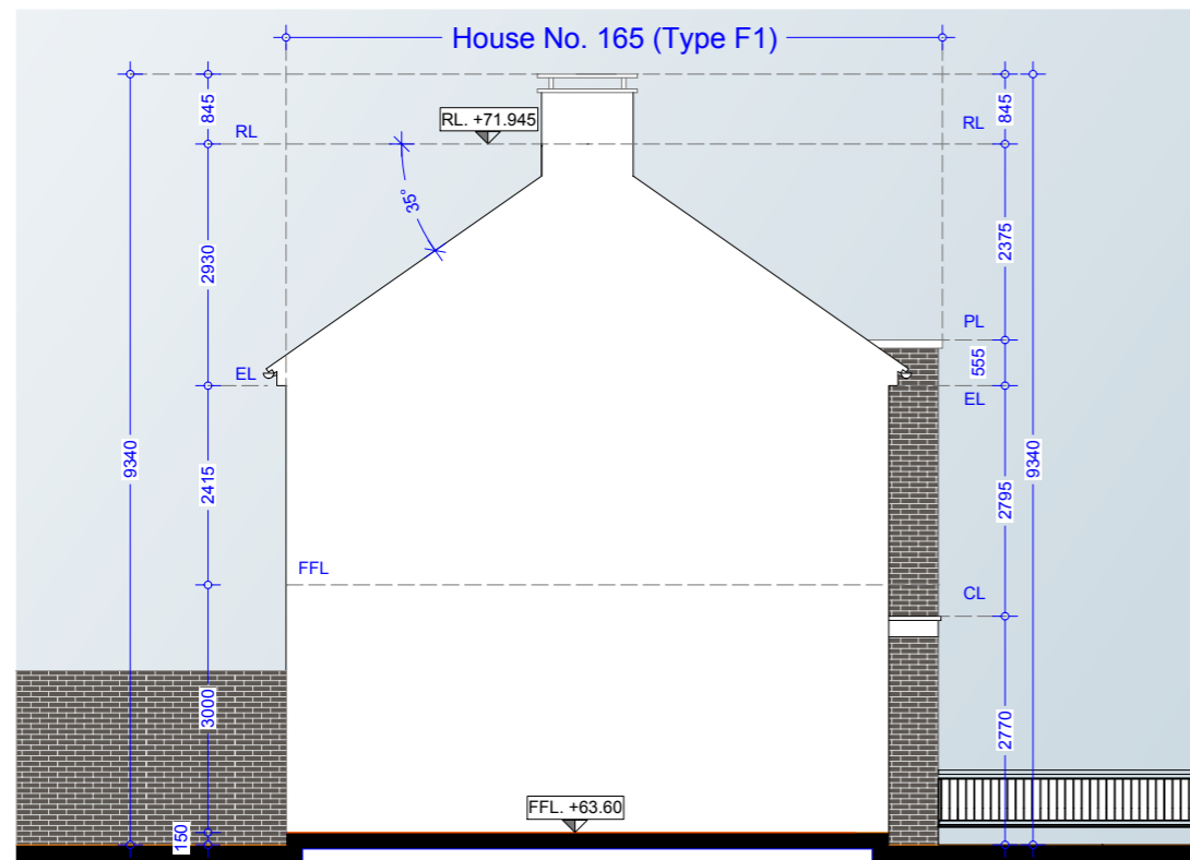
Side Elevation 01 - House Type F1
