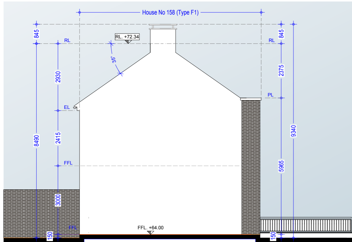
Side Elevation 01 - House Type F1
