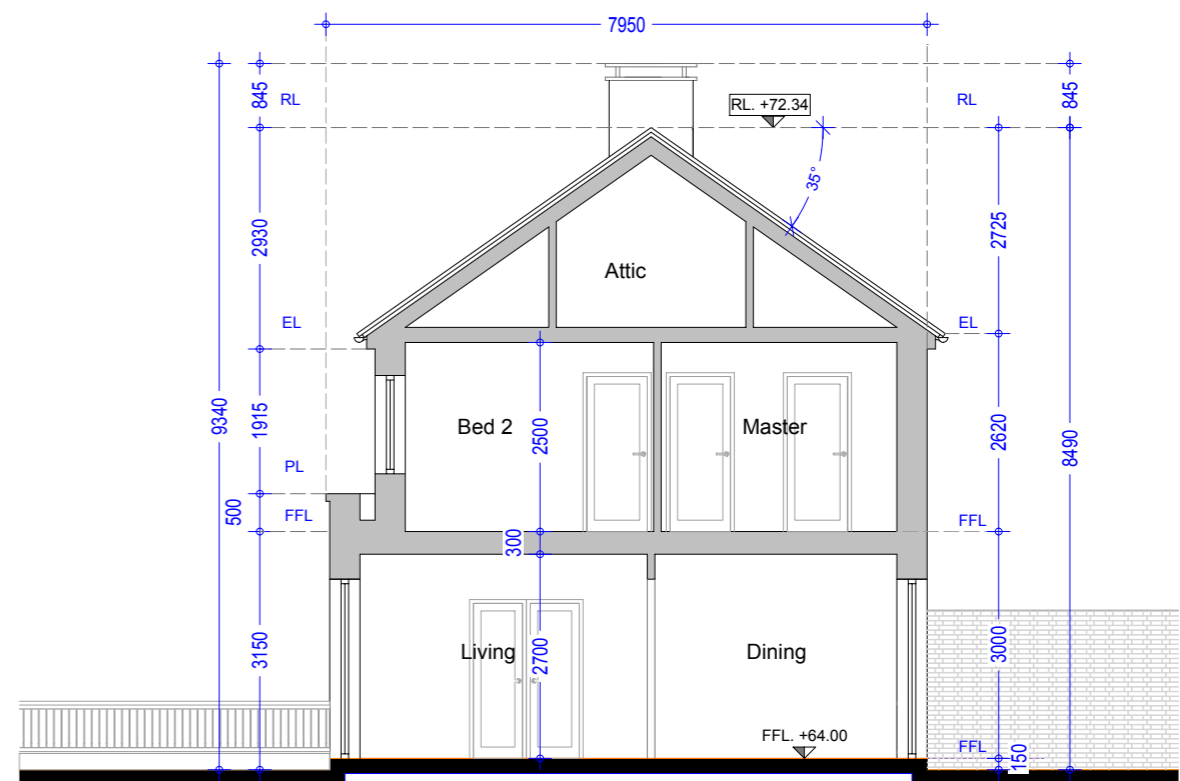
Section B-B - House No. 160 - Type E1
