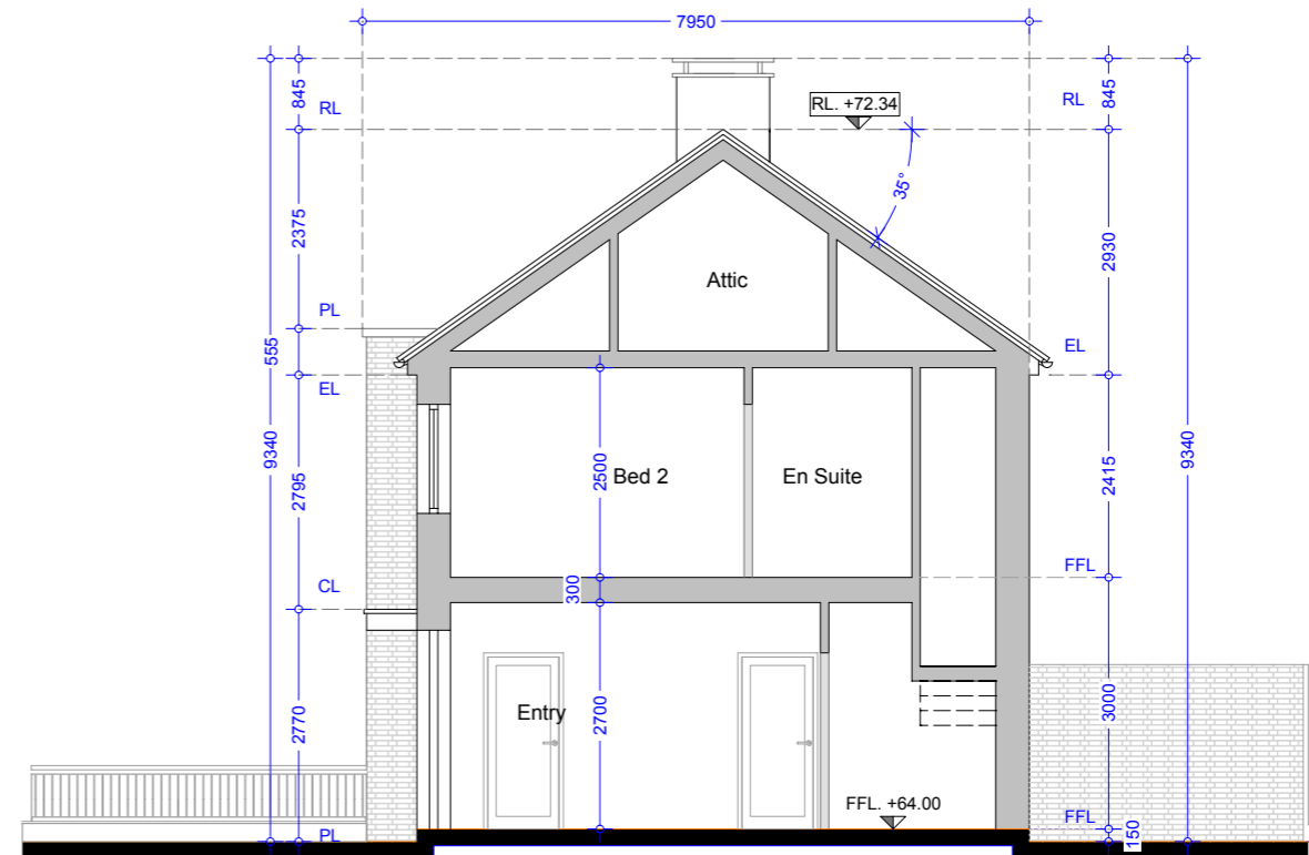
Section A-A - House No. 159 - Type F1
