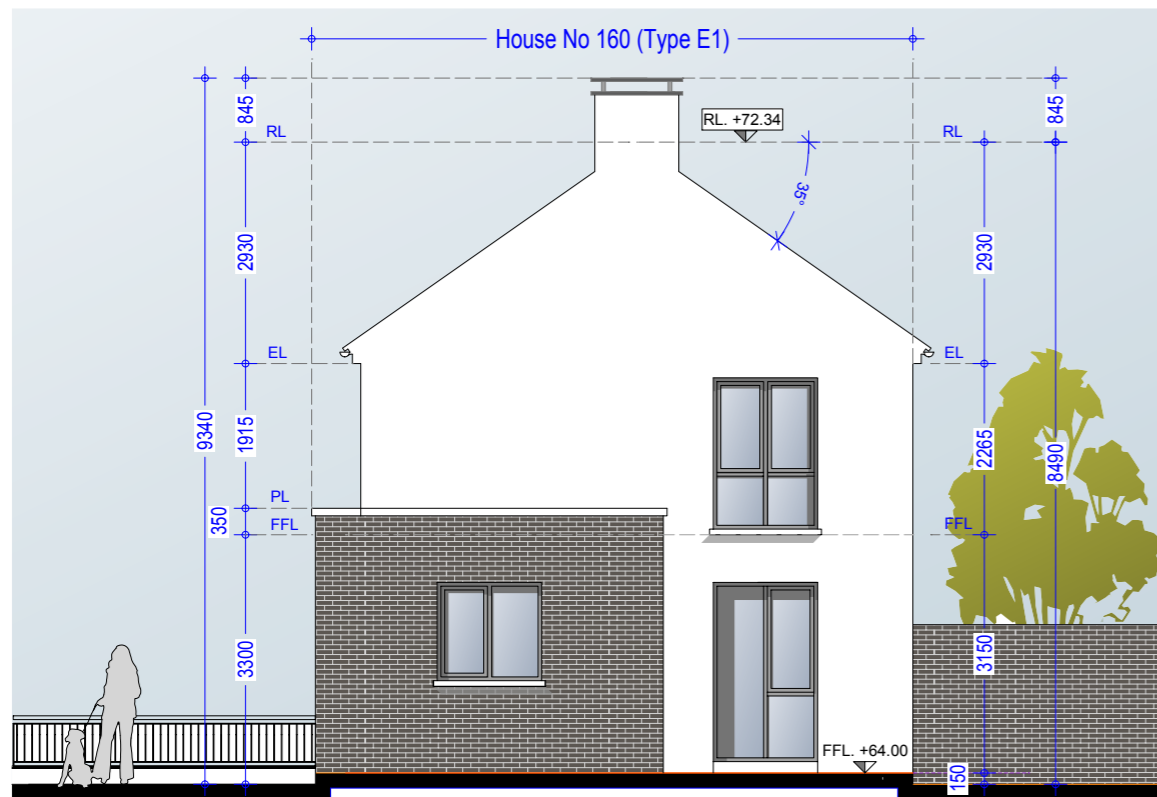
Side Elevation 02 - House Type E1
